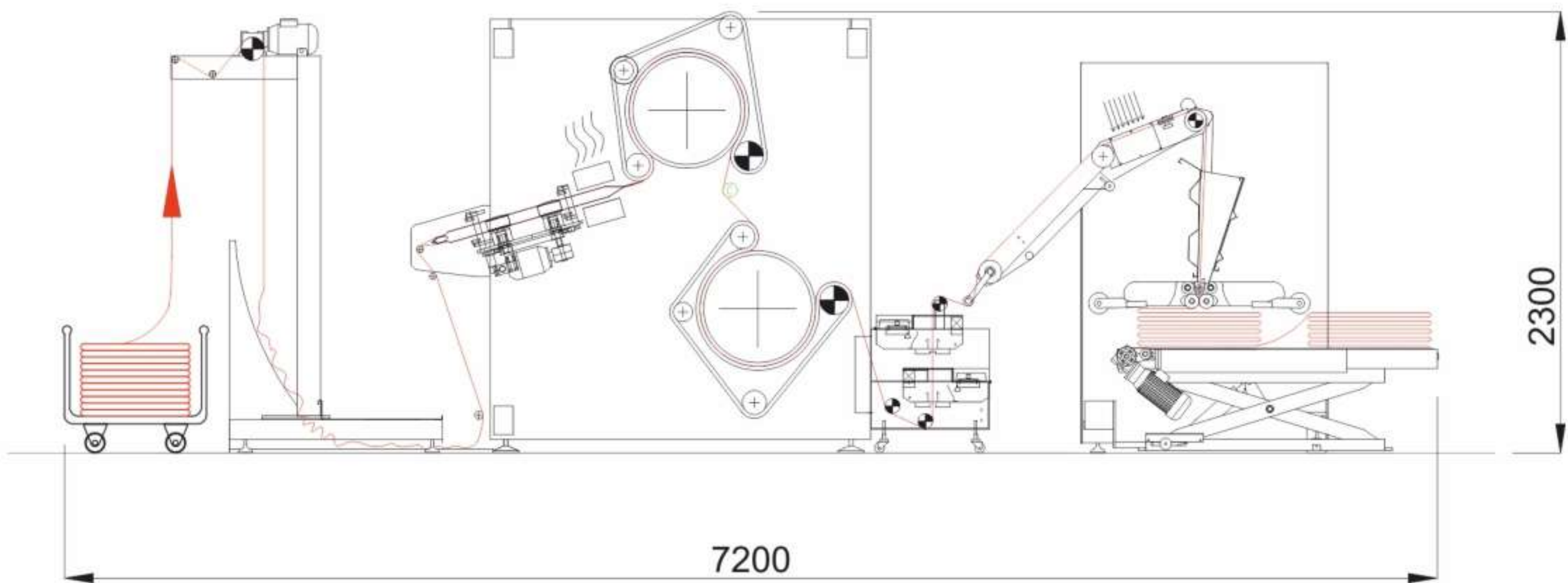
Tubular Felt Compactor + Dampening Unit (Felt Out) Tüp Keçeli Sanfor + Nemlendirme Ünitesi (Keçe Çıkışı)
