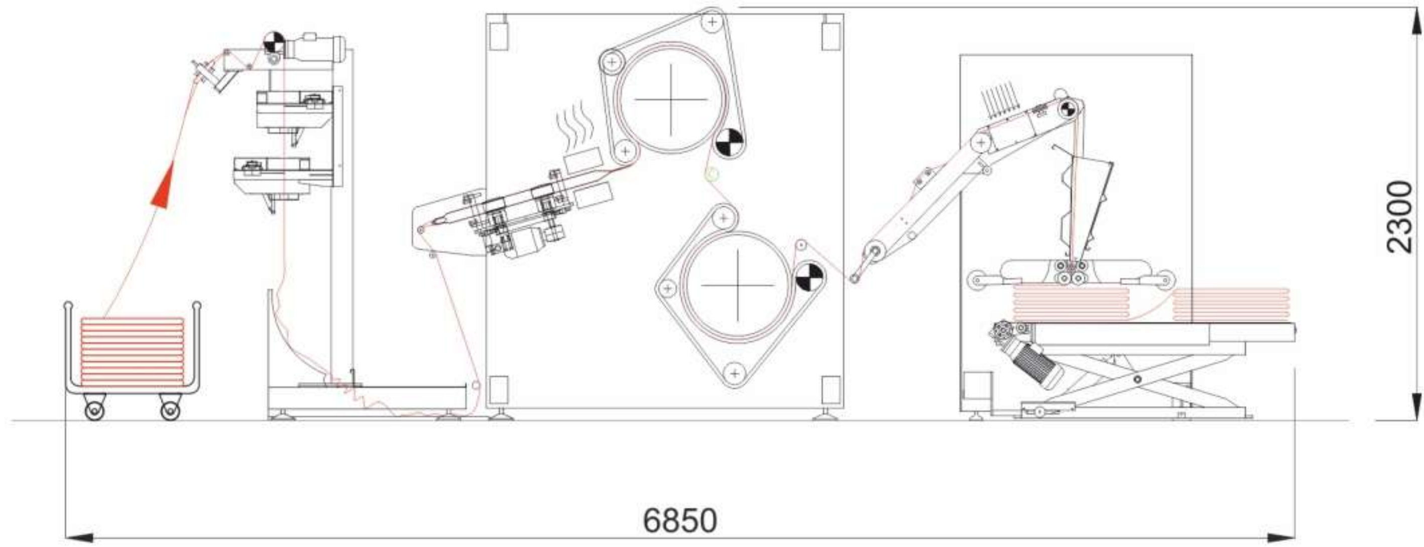
Tubular Felt Compactor + Dampening Unit (J-Box) Tüp Keçeli Sanfor + Nemlendirme Ünitesi (J-Box)
